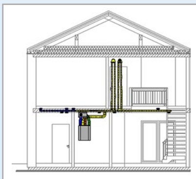
Abbildung 6: Darstellung Gebäudeschnitt
